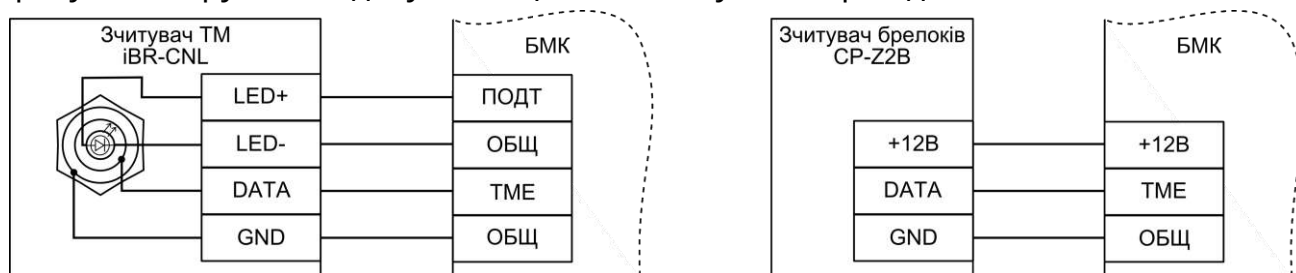
Рисунок 4 - Схема підключення зчитувача ключів ТМ (зліва) та зчитувача Proximity брелоків (зправа)
