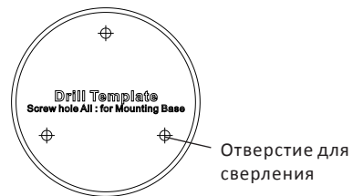
Рисунок 2-4 Шаблон крепления
