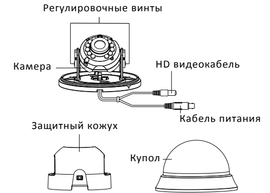
Рисунок 1-3 Камера III типа
