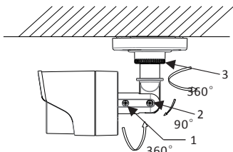
Рисунок 2-3 3-х осевая установка
